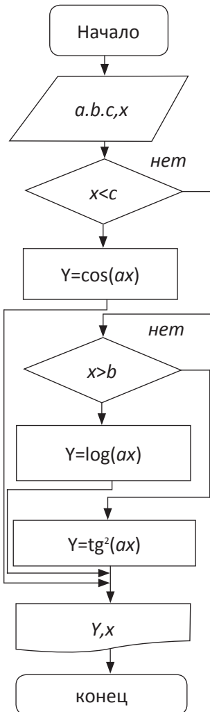
Рис. 3. Блок-схема алгоритма с двумя разветвлениями
